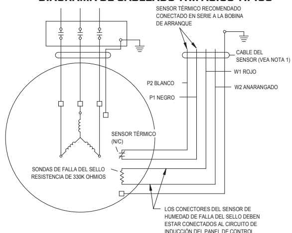
DIAGRAMA DE CABLEADO TRIFÁSICO TÍPICO
