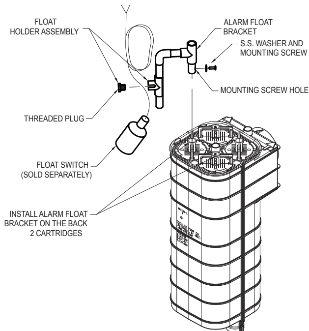
WW4 DELUXE EFFLUENT FILTER
