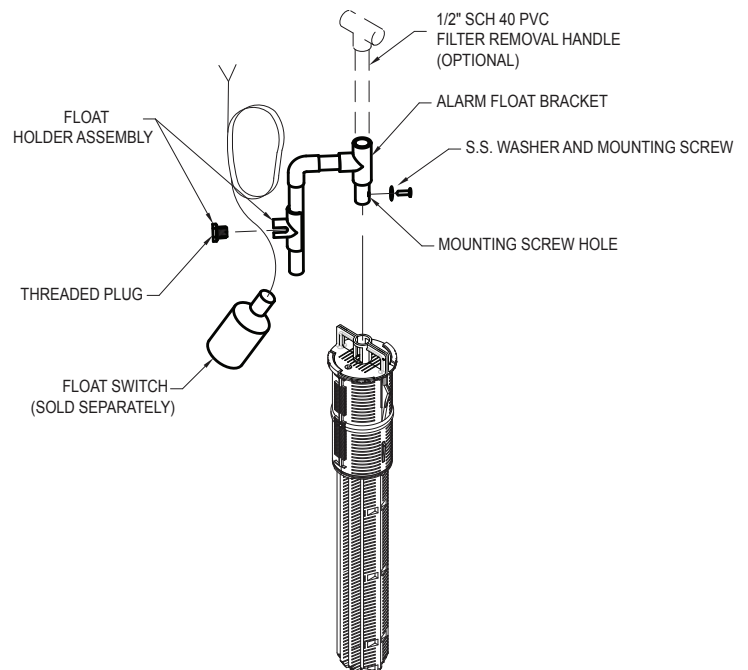
WW1 EFFLUENT FILTER
