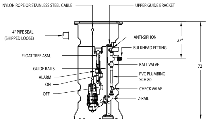
Z-Rail® shown
